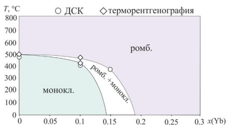
Рисунок 3—Схема полиморфного перехода в \text{Ca}_{3-1.5x}\text{Yb}_x\square_{0.5x}\text{B}_2\text{SiO}_8
