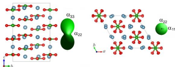
Рисунок 7 – Кристаллическая структура Ca 3 B 2 O 6 и фигуры тензора термического расширения
