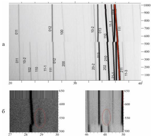
Рисунок 6 - а – Дифракционная картина \text{Ca}_2\text{V}_2\text{O}_5 в интервале температур 25–1010 °С, б – фрагменты дифракционной картины в интервалах температур 27–30 и 46–50°С.
