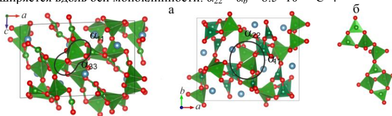
Рисунок 10– Кристаллическая структура бората \alpha\text{-CaV}_4\text{O}_7 в двух проекциях (а) и его полианион (б)
