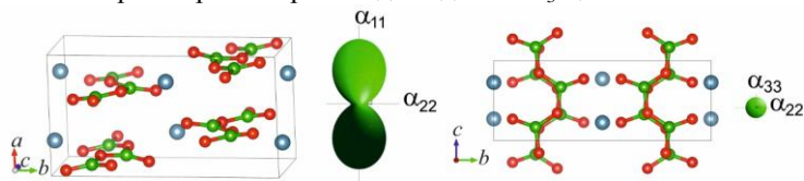
Рисунок 9 – Кристаллическая структура \text{CaV}_2\text{O}_4 и фигуры тензора термического расширения
